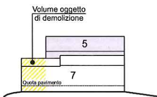
PROSPETTO EST
