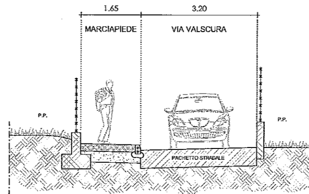
SEZIONE 5 - scala 1:100
