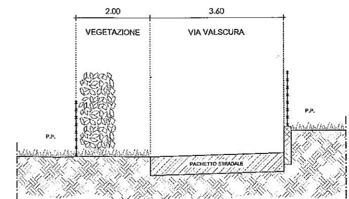
SEZIONE 8 - scala 1:100
