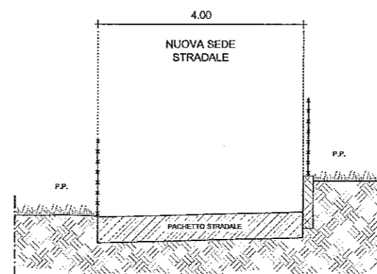
SEZIONE 7 - scala 1:100
