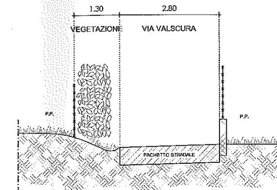
SEZIONE 6 - scala 1:100
