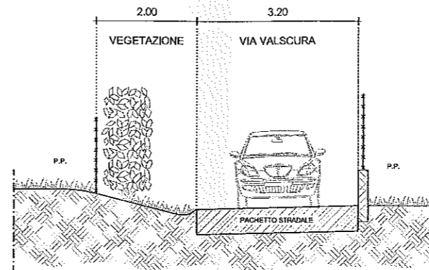
SEZIONE 5 - scala 1:100
