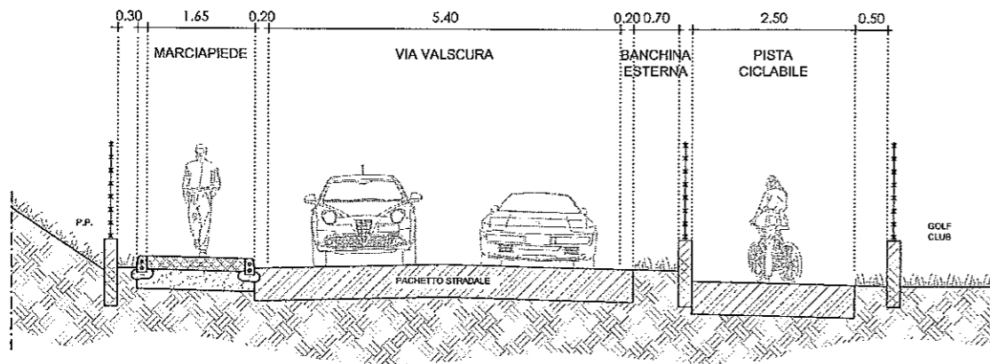
SEZIONE 2 - scala 1:100
