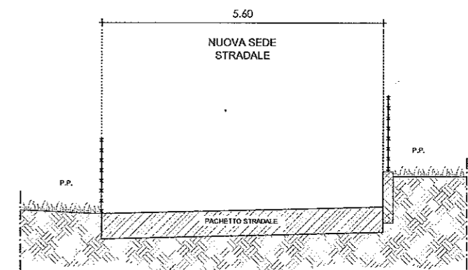
SEZIONE 8 - scala 1:100
