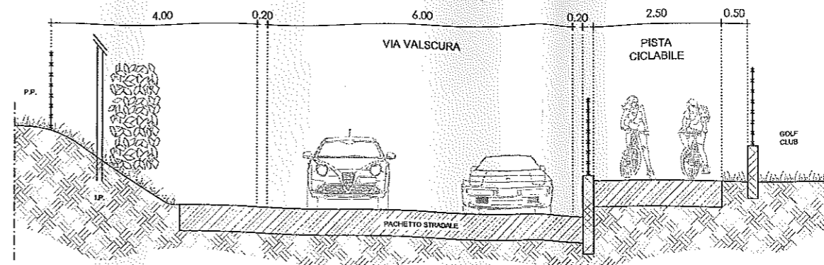
SEZIONE 4 - scala 1:100
