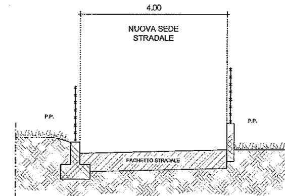
SEZIONE 6 - scala 1:100
