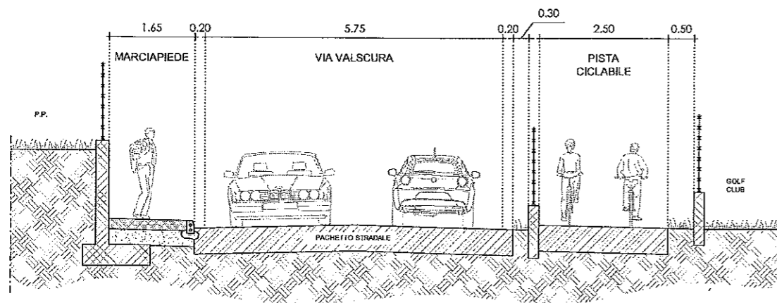
SEZIONE 3 - scala 1:100
