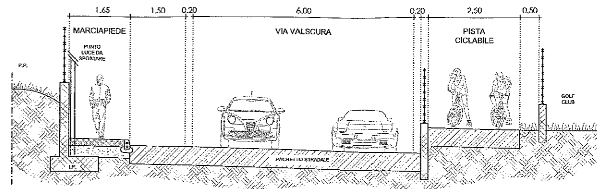
SEZIONE 4 - scala 1:100
