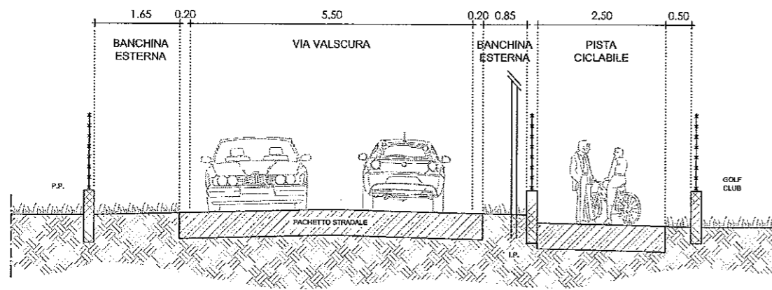
SEZIONE 1 - scala 1:100
