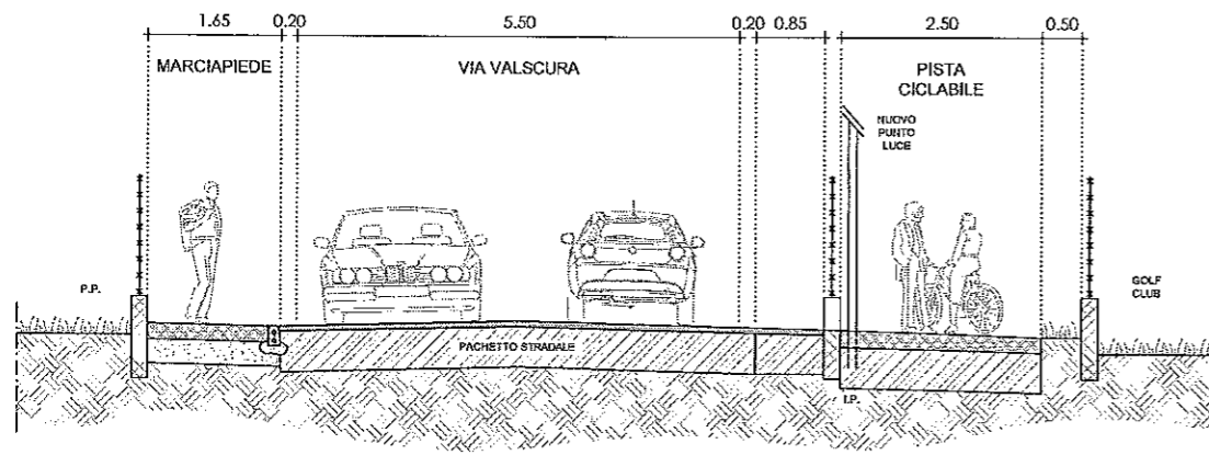
SEZIONE 1: attraversamento pedonale- scala 1:100
