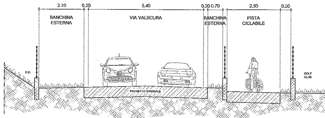
SEZIONE 2 - scala 1:100
